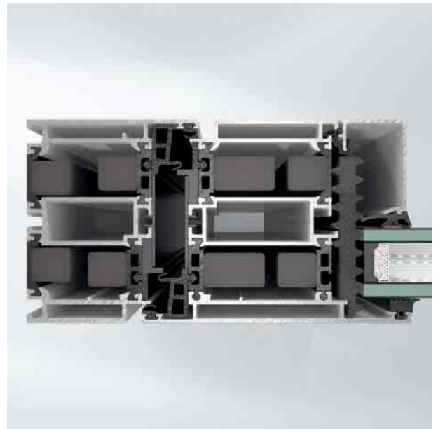
Schüco Tür ADS 90.SI SimplySmart Schüco Door ADS 90.SI SimplySmart
