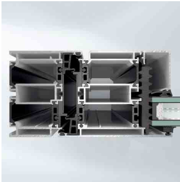
Schüco Tür ADS 90 SimplySmart Schüco Door ADS 90 SimplySmart
